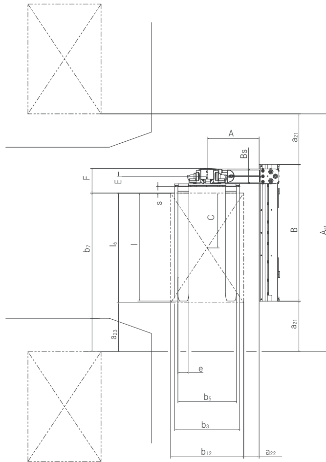
Fourche tridirectionnelle - vue de dessus
