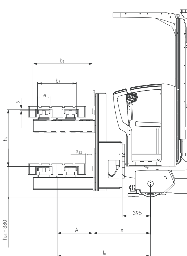
MX-X avec fourche télescopique haute - vue de coupe
