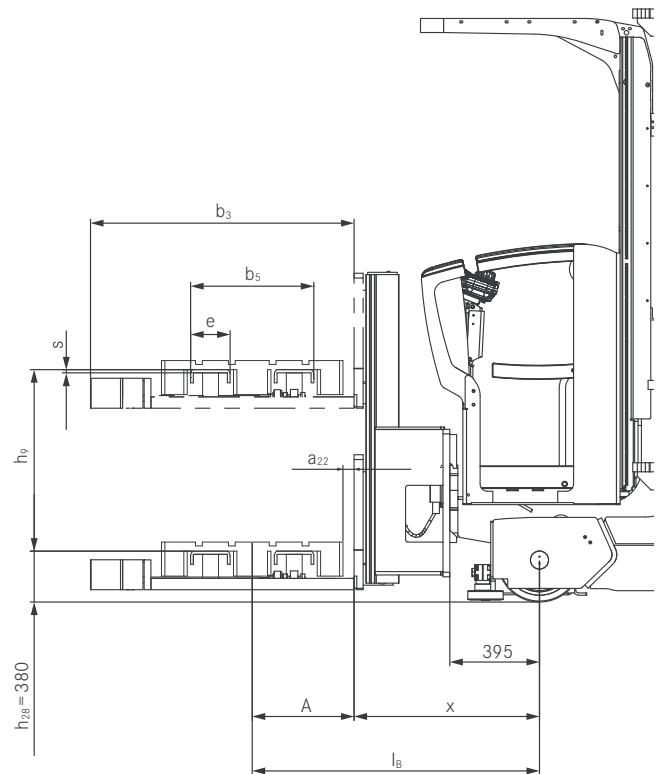
MX-X avec fourche télescopique basse - vue de coupe
