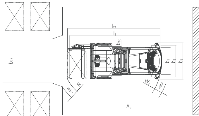
MX-X avec fourche tridirectionnelle et guidage mécanique - vue de dessus
